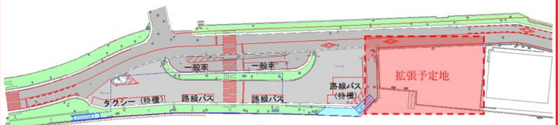
計画平面図
